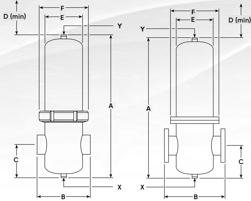
Dişli BSP ve NPT
